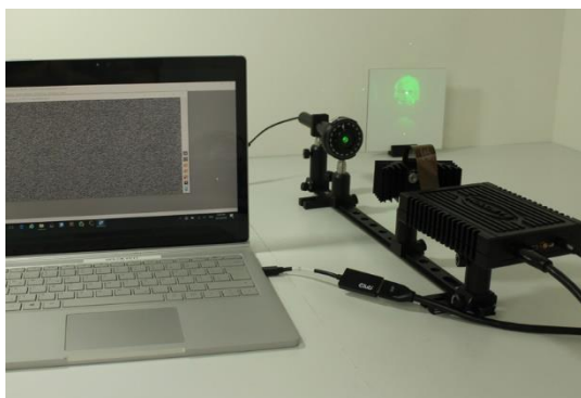
Obr. 1: Spatial light modulator, zdroj: Holoeye
